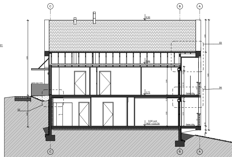
B Coupe BB
