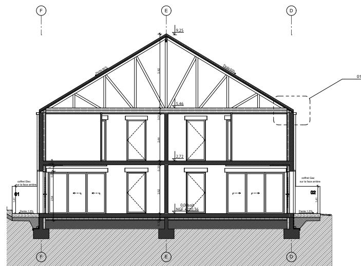
A Coupe AA
